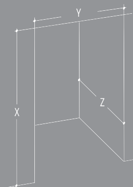
Vano incasso
