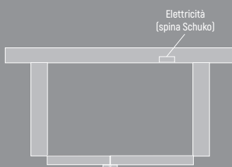
Schema installazione
