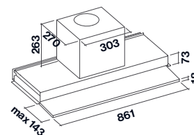
Vista laterale con camini opzionali
