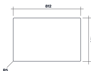
Dimensioni foro per installazione in appoggio
