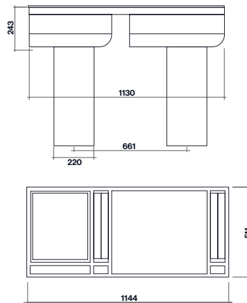
Modula/M3: Piastra teppanyaki + Piano induzione 60 cm
