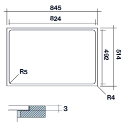
Dimensioni foro per installazione a filo (M1/M2)
