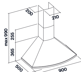
Versione parete
