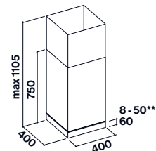
Versione parete telescopica **Risiega regolabile.
