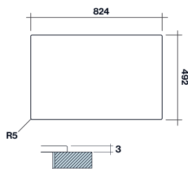
Dimensioni foro per installazione in appoggio (M1/M2)
