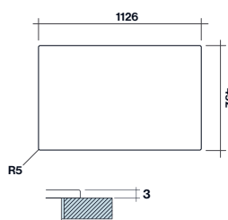
Dimensioni foro per installazione in appoggio (M3)
