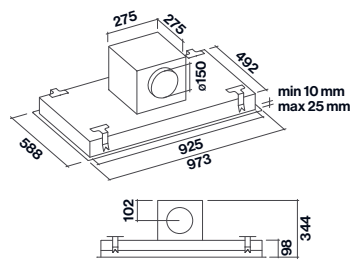
Motore sottotetto installato sulla cappa
