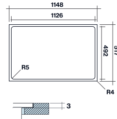
Dimensioni foro per installazione a filo (M3)
