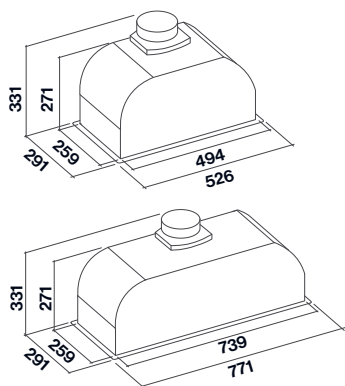
Foro per incasso 50 cm: 506 mm x 262 mm 70 cm: 751 mm x 262 mm
