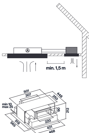
Foro per incasso 533 mm x 434 mm
