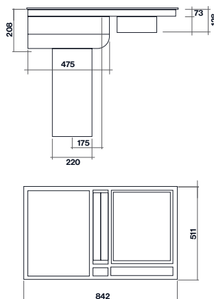
Modula/M2: Piastra teppanyaki + Piano induzione 38 cm
