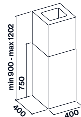
Versione isola
