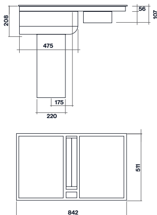
Modula/M1: Piano induzione 38 cm x 2
