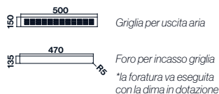
Foro per incasso 470 mm x 135 mm
