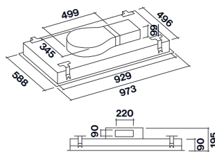
Motore Slim (solo su cappa)
