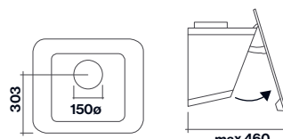
Vista posteriore
