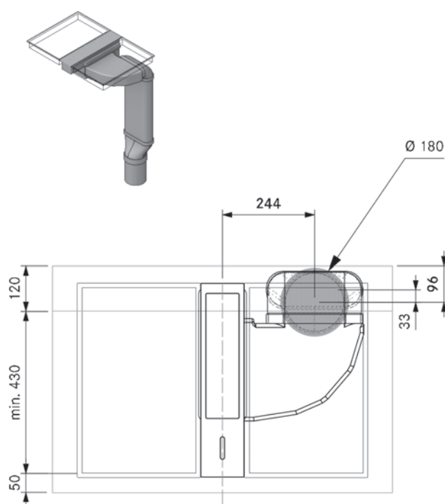
CKA2 con canale piatto EFS750, riduttore diritto EFRG e silenziatore in cantina
