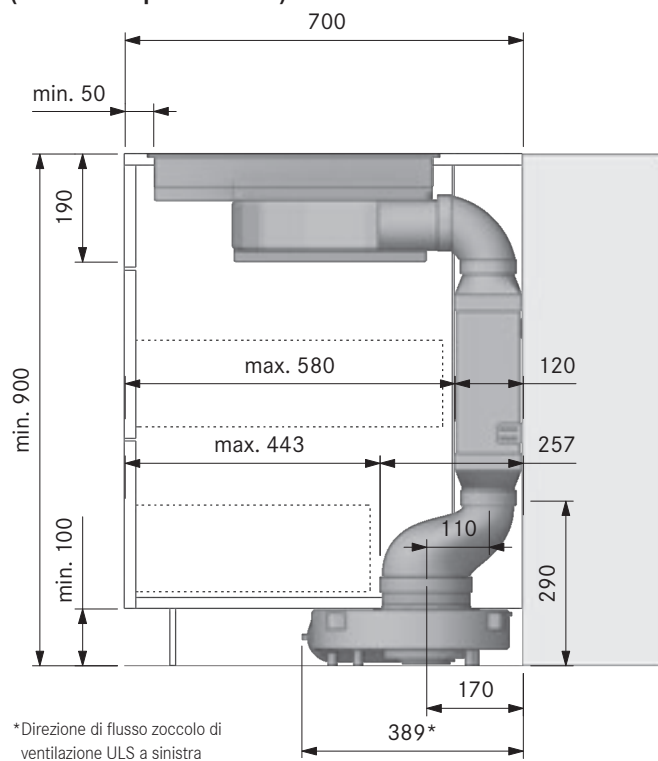
Intaglio vano incasso CKA2 con silenziatore piatto USDF + riduttore passaggio piatto rotondo sfasato EFRV110/1 (cucina componibile 700):
