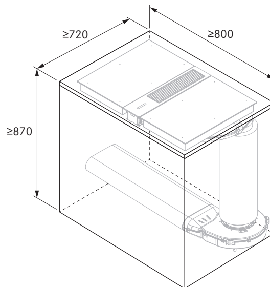
Dimensione minima vano incasso CKA2 + USDR50:
