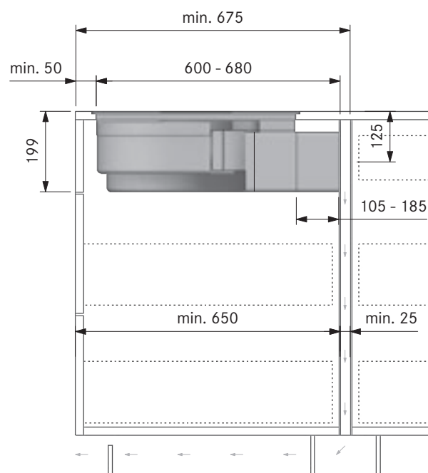
Intaglio vano incasso PURU + PULBTA (cucina a isola):
