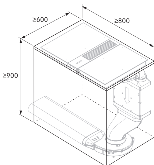
Dimensione minima vano incasso CKA2 (Caso speciale):
