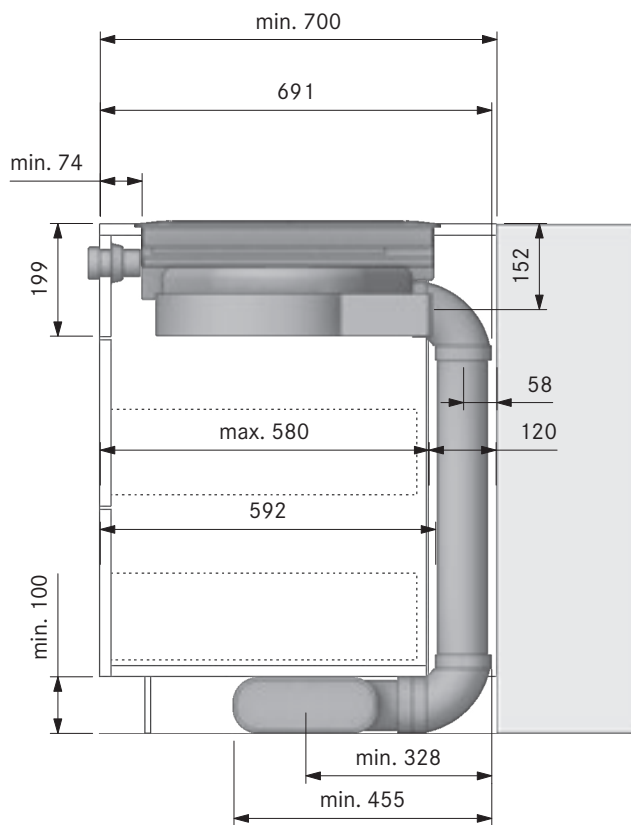
Intaglio vano incasso PKA con Ecotube canale piatto:
