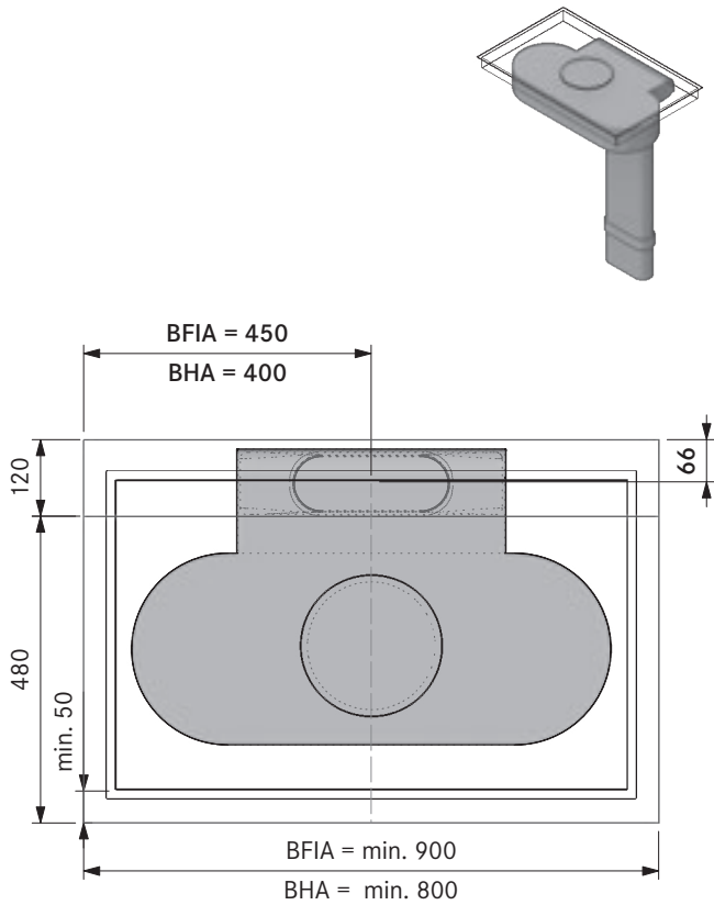
Dimensione minima preforo Basic + EF750 (cucina componibile 600):
