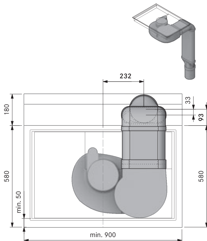
Dimensione minima preforo PUXA + EF750 + EFRG (cucina a isola):
