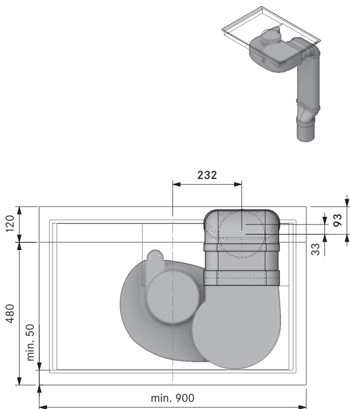
Dimensione minima preforo PUXA + EF750 + EFRG (cucina componibile):
