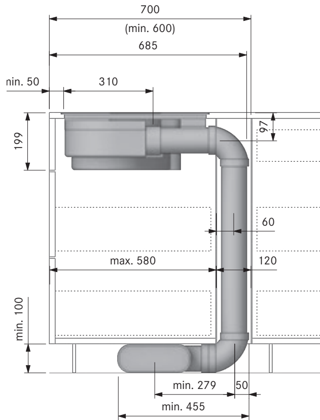
Intaglio vano incasso PURA (cucina a isola):
