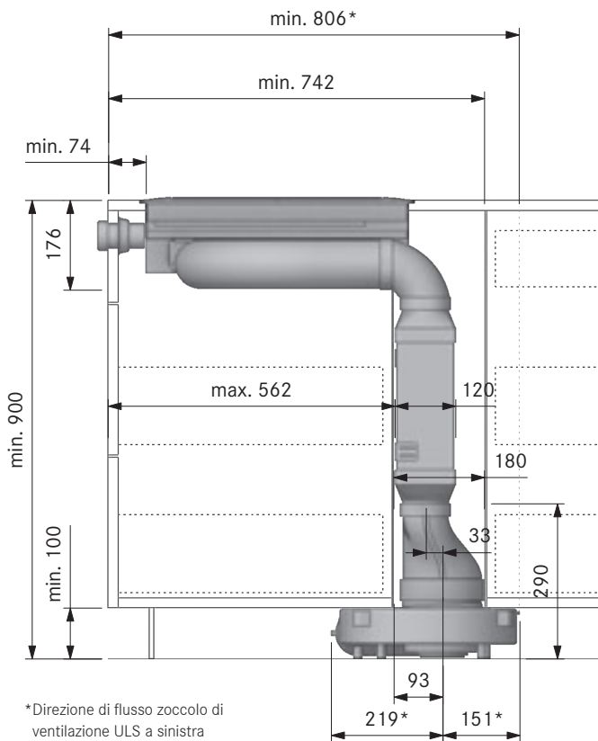
Intaglio vano incasso PKA con silenziatore piatto USDF e riduttore dritto EFRG (cucina a isola):
