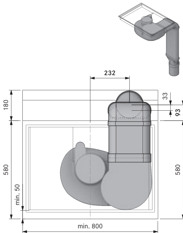
Dimensione minima preforo PURA + EF750 + EFRG (cucina a isola):
