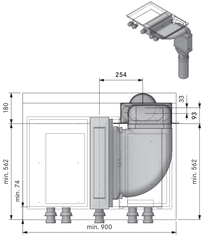
Dimensione minima preforo PKA + USDF + EFRG (cucina a isola):
