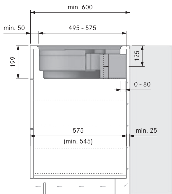
Intaglio vano incasso PURU (cucina componibile 600):
