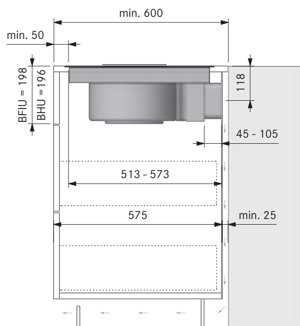
Intaglio vano incasso Basic funzionamento filtrante (cucina componibile 600):
