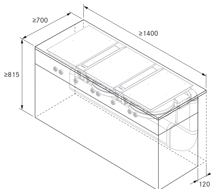
Dimensione minima vano incasso 2 PKAS (sistema di scarico aria):
