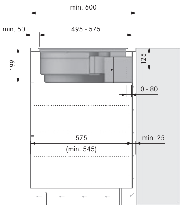
Intaglio vano incasso PUXU (cucina componibile 600):
