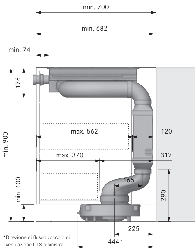
Intaglio vano incasso PKA con silenziatore piatto USDF e riduttore sfasato EFRV (cucina componibile):
