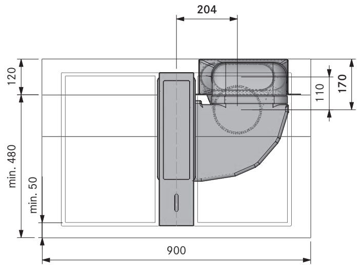
Dimensione minima preforo CKA2 + EF750 + EFRG:
