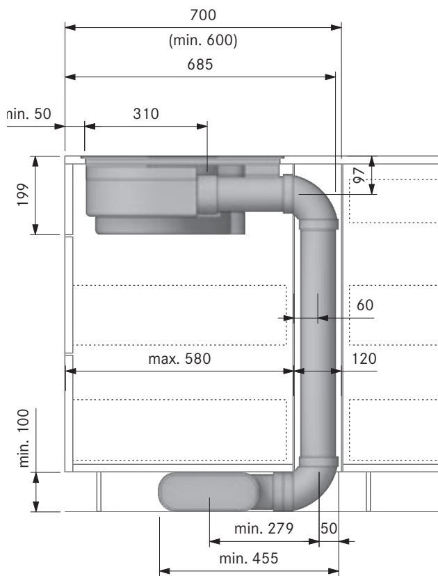
Intaglio vano incasso PUXA (cucina a isola):
