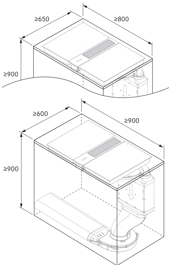
Dimensione minima vano incasso CKA2 + USDF (Dimensioni comfort 800x650 mm e 900x600 mm):
