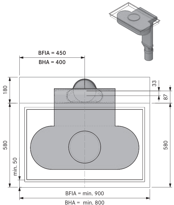
Dimensione minima preforo Basic + EF750 + EFRG (cucina a isola):
