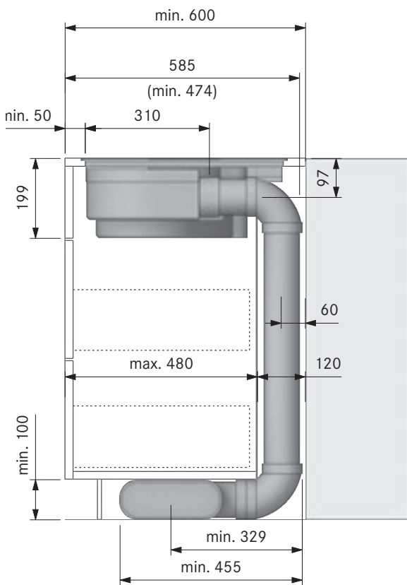
Intaglio vano incasso PUXA (cucina componibile 600):
