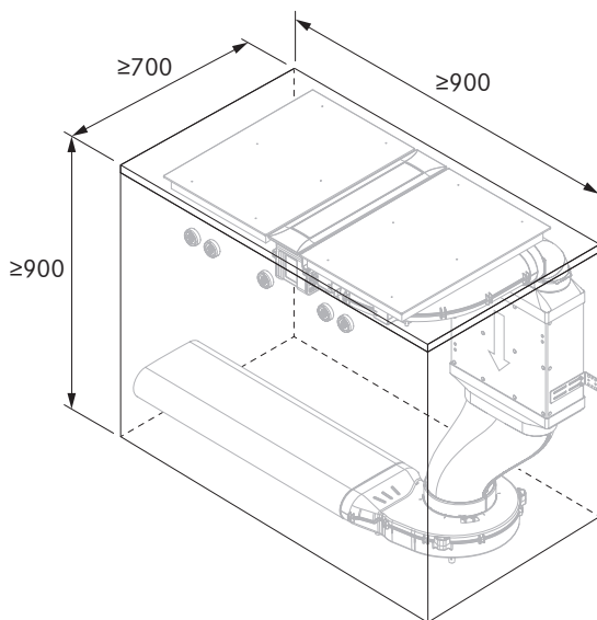
Dimensione minima vano incasso PKA + PESDF:
