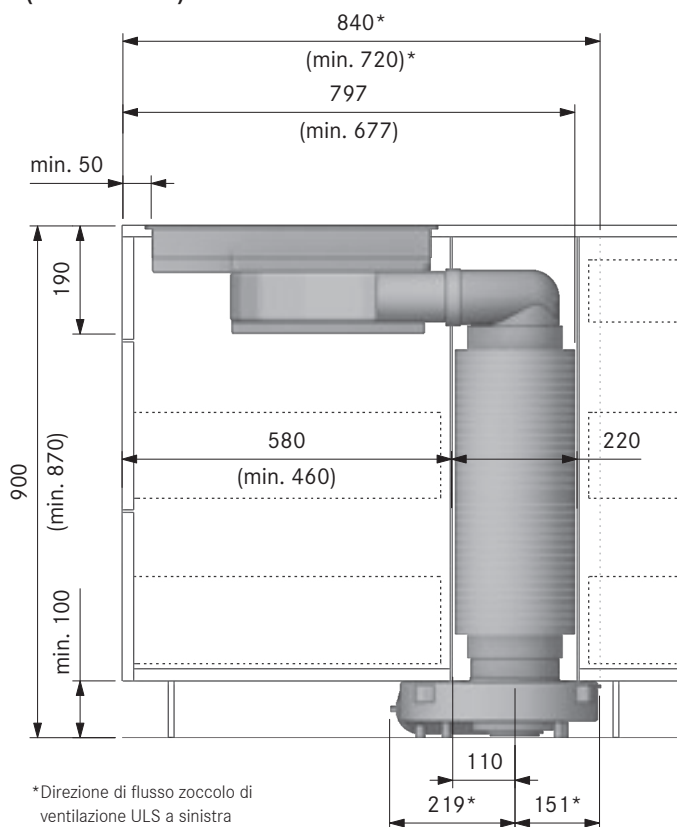
Intaglio vano incasso CKA2 con silenziatore rotondo USDR50 (cucina a isola):
