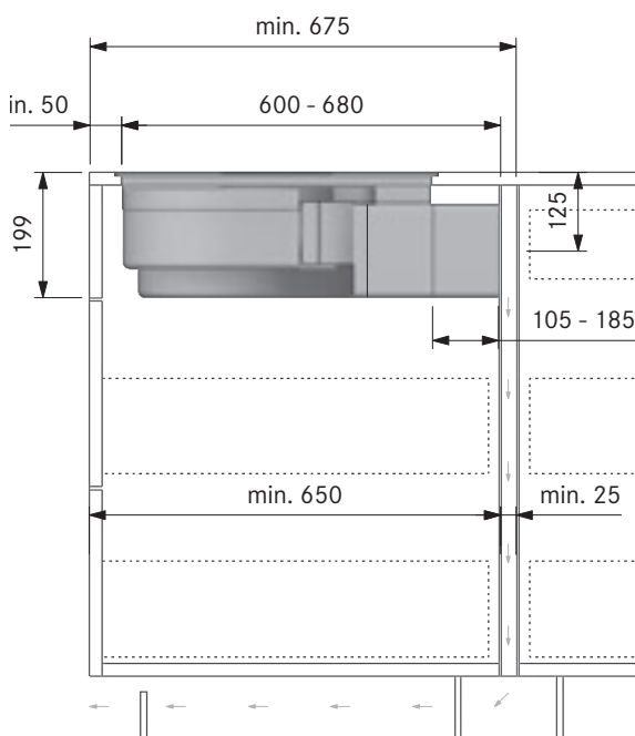
Intaglio vano incasso PUXU + PULBTA (cucina a isola):
