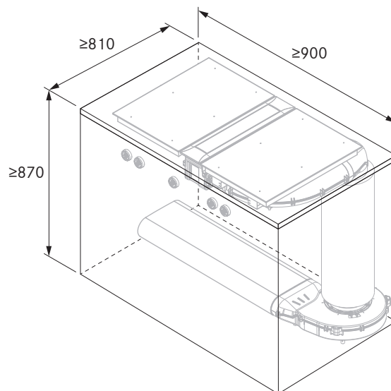
Dimensione minima vano incasso PKA + PESDR:
