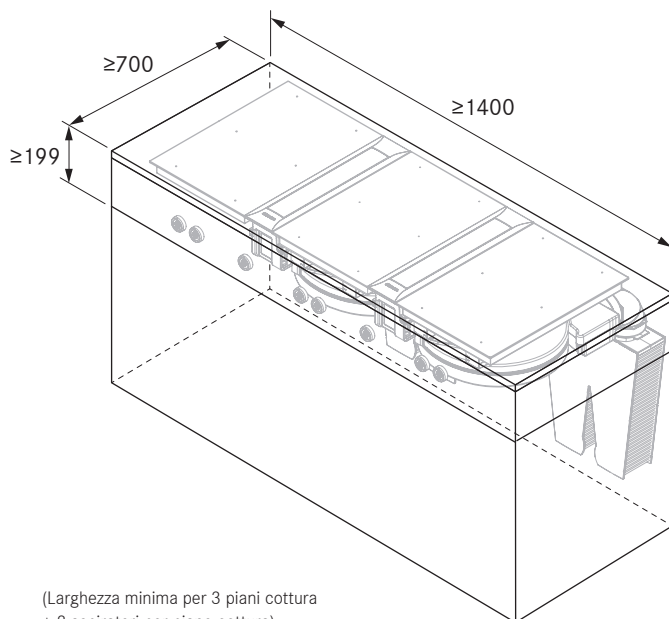
Dimensione minima vano incasso 2 PKAS + 2 EFBV90 + 2 ULBF:
