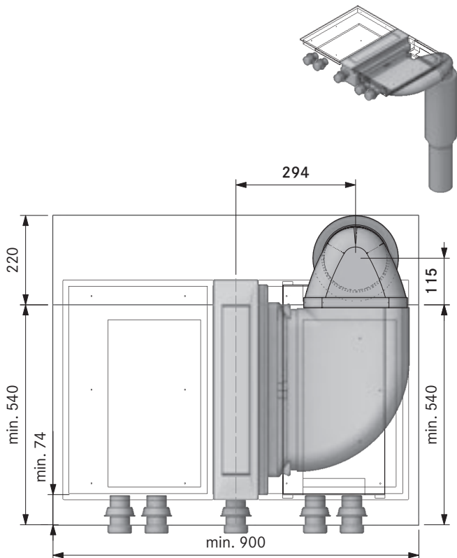
Dimensione minima preforo PKA + USDR50 (cucina a isola):
