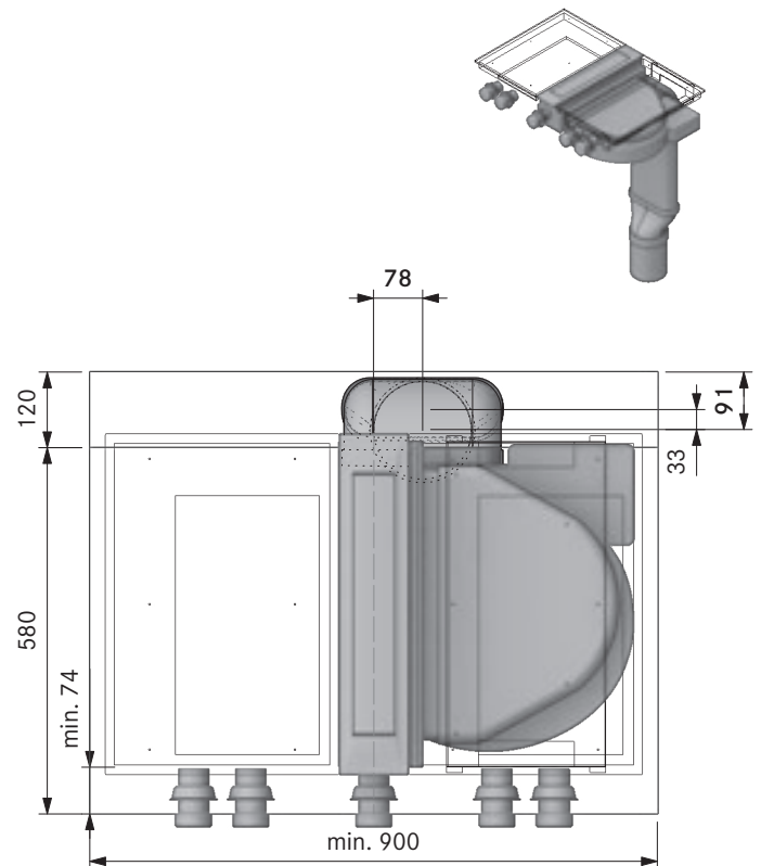
Dimensione minima preforo PKAS + EF750 + EFRG (cucina componibile):
