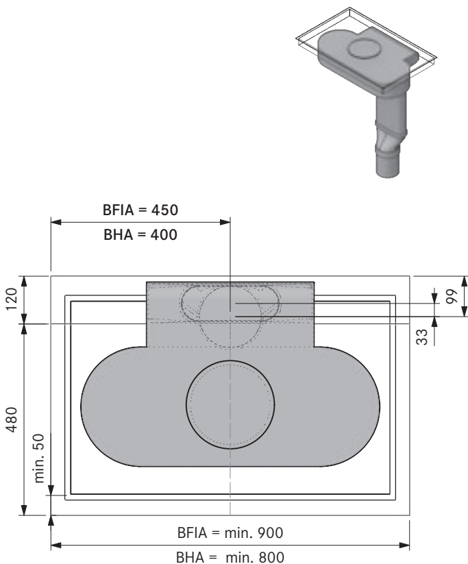
Dimensione minima preforo Basic + EF750 + EFRG (cucina componibile):
