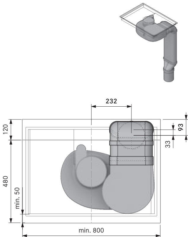
Dimensione minima preforo PURA + EF750 + EFRG (cucina componibile):
