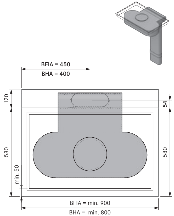
Dimensione minima preforo Basic + EF750 (cucina a isola 700):
