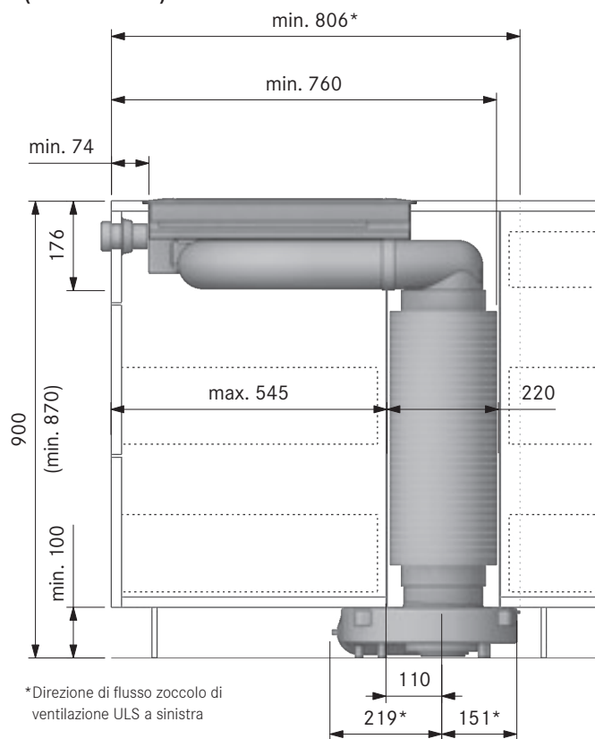
Intaglio vano incasso PKA con silenziatore rotondo USDR50 (cucina a isola):
