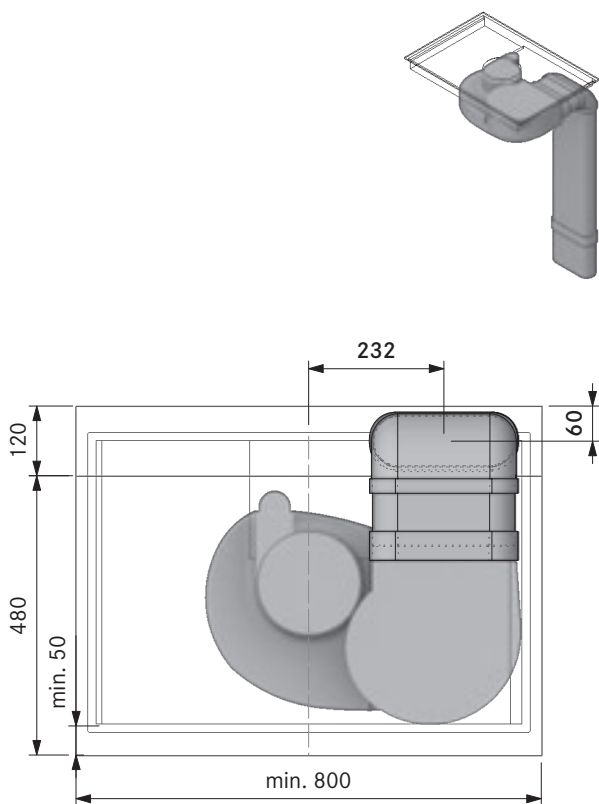
Dimensione minima preforo PURA + EF750 (cucina componibile 600):
