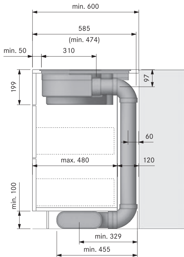
Intaglio vano incasso PURA (cucina componibile 600):
