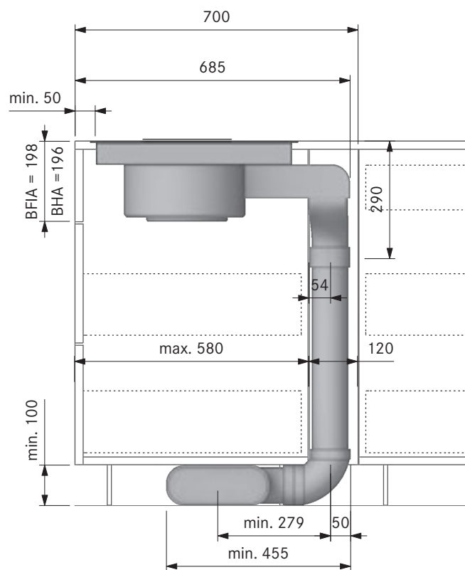
Intaglio vano incasso Basic aspirante (cucina a isola 700):
