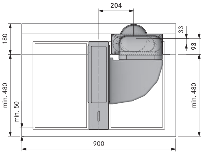
Dimensione minima preforo CKA2 + USDR50 (cucina a isola):
