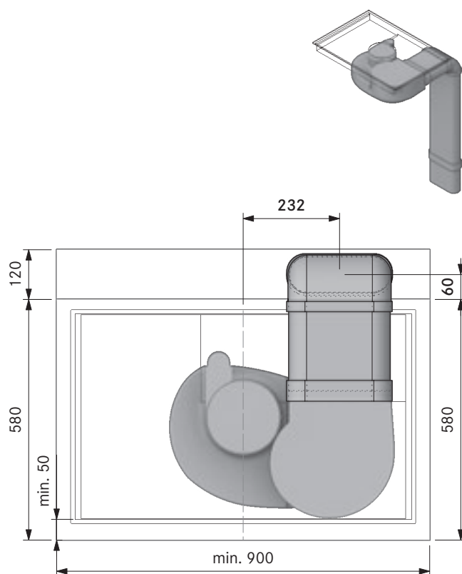
Dimensione minima preforo PUXA + EF750 (cucina a isola 700):
