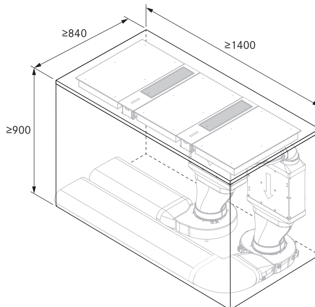
Dimensione minima vano incasso 2 CKA2 + 2 USDF:
