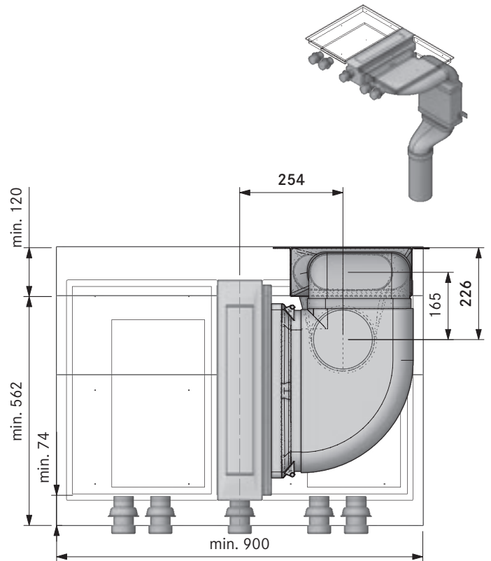
Dimensione minima preforo PKA + USDF + EFRV (cucina componibile):
