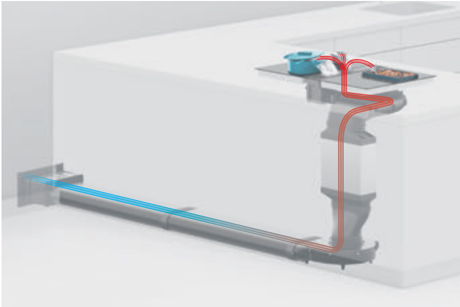
Esempio di montaggio aria di scarico BORA Classic 2.0 – CKA2 (stesso principio per Professional, X Pure, Pure e Basic)
