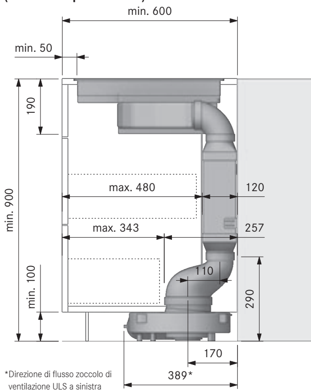
Intaglio vano incasso CKA2 con silenziatore piatto USDF + riduttore passaggio piatto rotondo sfasato EFRV110/1 (cucina componibile 600):
