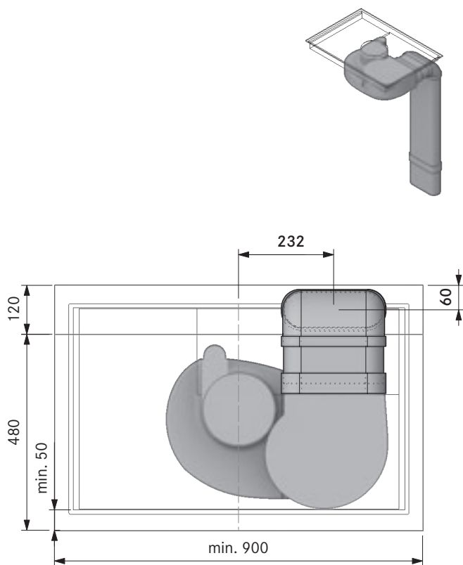
Dimensione minima preforo PUXA + EF750 (cucina componibile 600):
