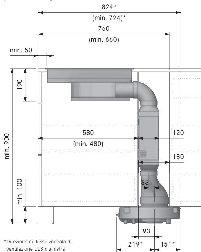
Intaglio vano incasso CKA2 con silenziatore piatto USDF + riduttore piatto rotondo dritto EFRG/1 (cucina a isola):
