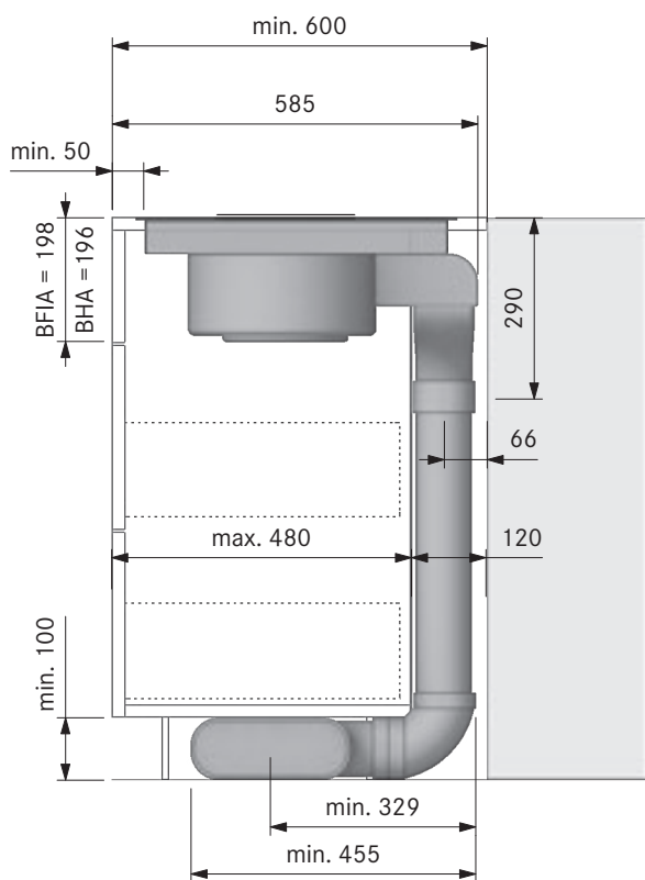
Intaglio vano incasso Basic aspirante (cucina componibile 600):
