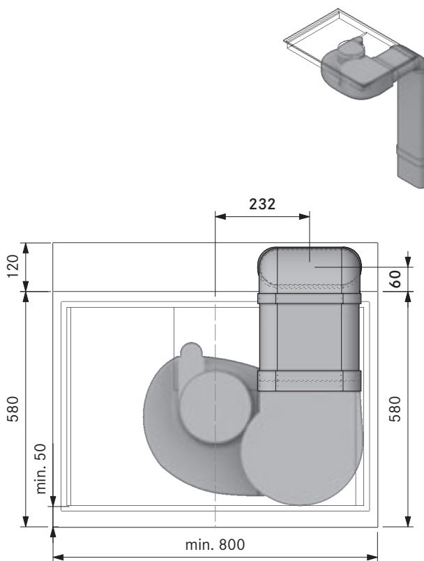
Dimensione minima preforo PURA + EF750 (cucina a isola 700):
