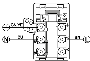
220-240V 1N ~
