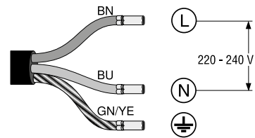
220-240V 1N ~
