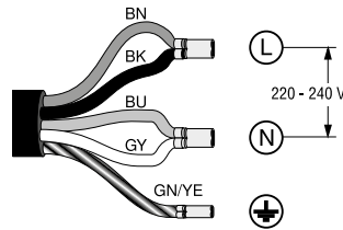
220-240V 1N ~
